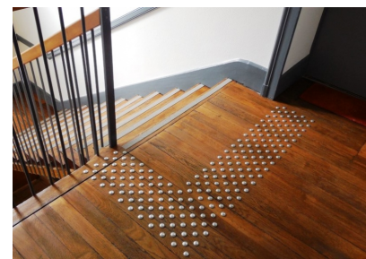
Détail : éléments podotactiles pour les personnes malvoyantes.
